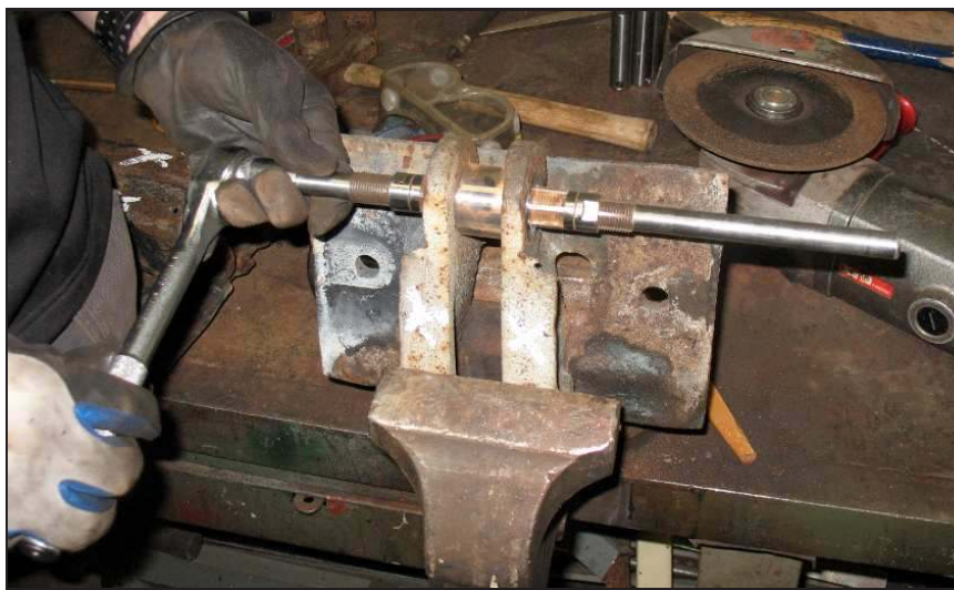
Brotskning av hål för bandbult i bandplatta
